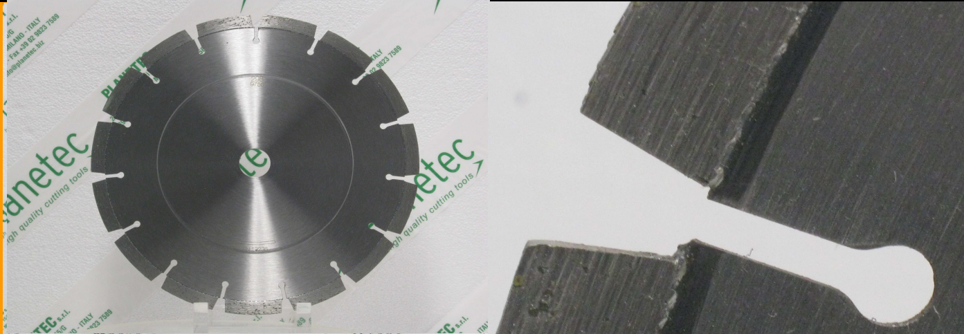
esempio di disco con segmento alto 10 mm - sample of disc with segment height 10 mm
